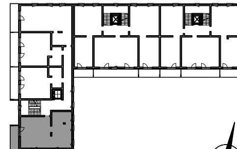
BUDYNEK B3 PRZY UL. OBROŃCÓW LUBLINA KLATKA 2 POZIOM 2
