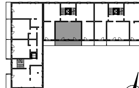
BUDYNEK B3 PRZY UL. OBRONCÓW LUBLINA KLATKA 2 POZIOM 2
